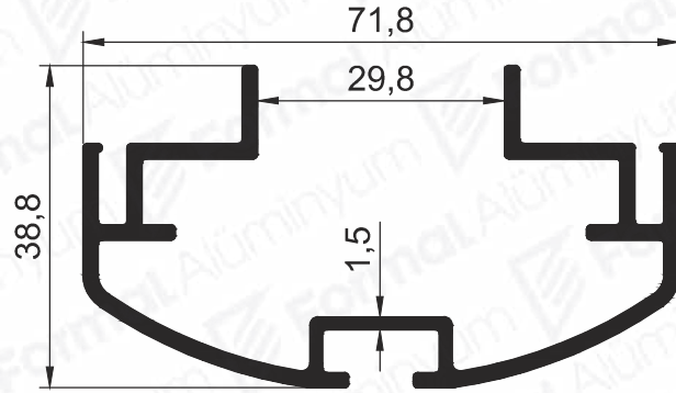
Pr.No: 8910 1,024 kg/m
