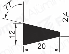
Pr.No: 9689 0,390 kg/m
