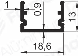
Pr.No: 4612 0,131 kg/m
