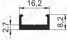
Pr.No: 9426 0,149 kg/m
