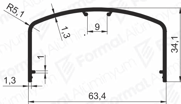
Pr.No: 8569 0,443 kg/m
