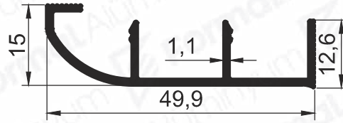
Pr.No: 2207 0,302 kg/m
