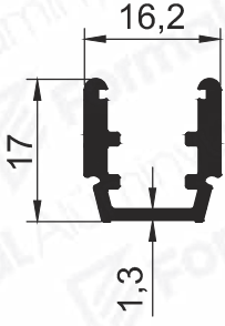
Pr.No: 9425 0,247 kg/m
