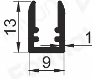
Pr.No: 1595 0,111 kg/m
