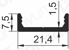
Pr.No: 2206 0,132 kg/m
