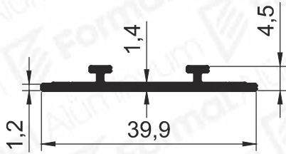
Pr.No: 4392 0,184 kg/m
