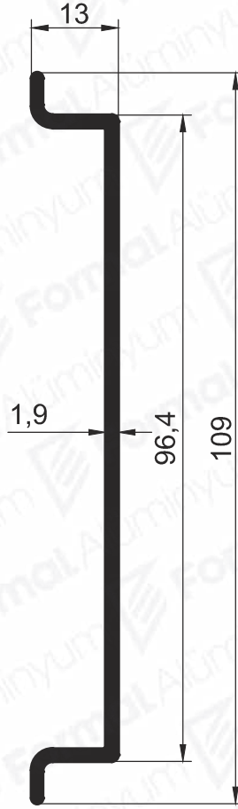
Pr.No: 9790 0,657 kg/m
