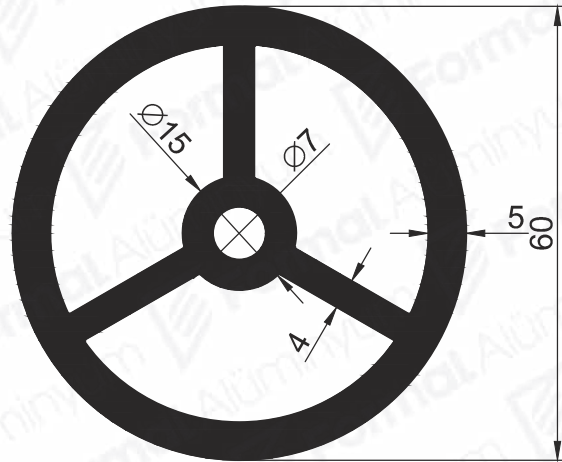
Pr.No: 8977 3,287 kg/m
