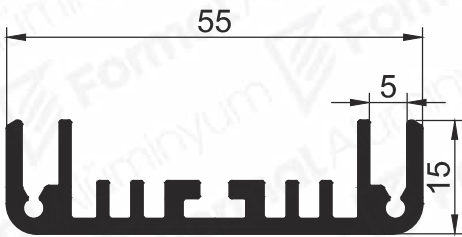
Pr.No: 9916 0,756 kg/m
