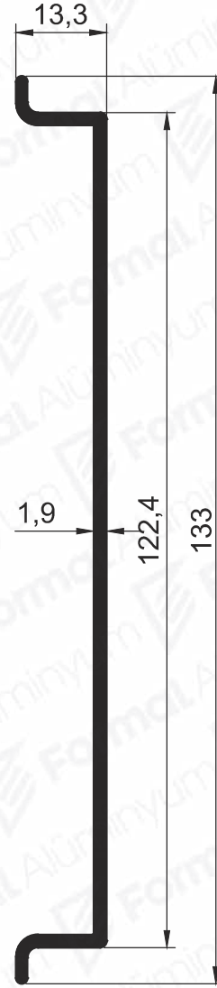
Pr.No: 9791 0,785 kg/m
