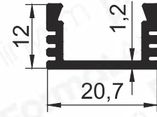
Pr.No: 2474 0,182 kg/m
