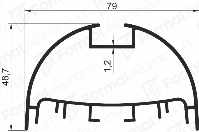
Pr.No: 8962 1,023 kg/m
