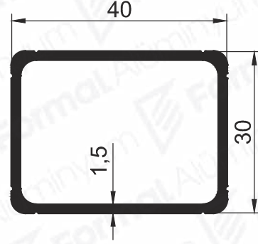
Pr.No: 3769 0,545 kg/m
