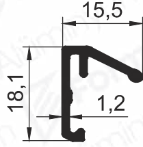
Pr.No: 3203 0,145 kg/m
