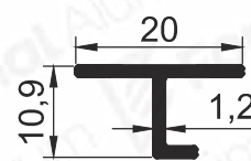
Pr.No: 8652 0,106 kg/m
