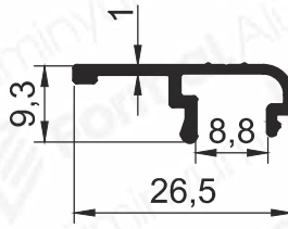
Pr.No: 8027 0,125 kg/m
