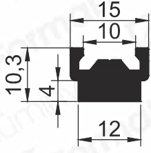
Pr.No: 1962 0,288 kg/m
