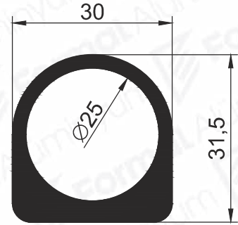
Pr.No: 8527 0,955 kg/m
