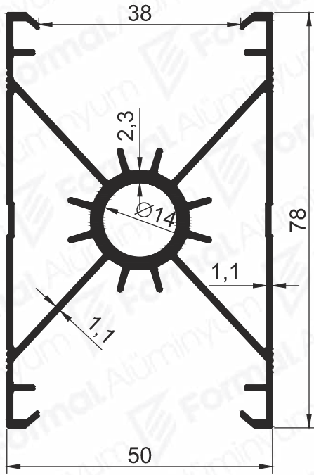
Pr.No: 1959 2,031 kg/m
