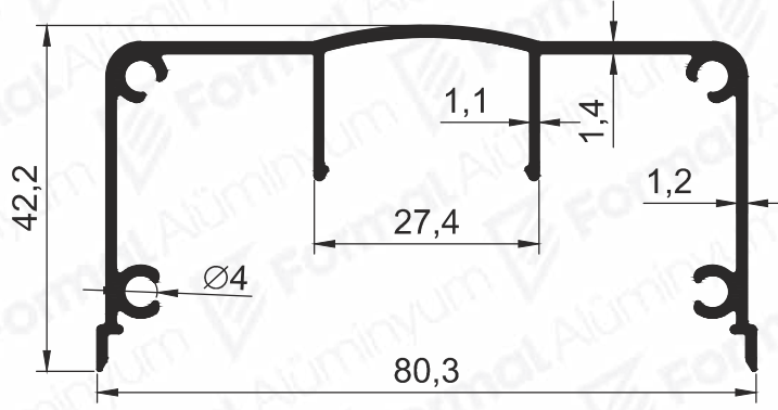
Pr.No: 1723 0,804 kg/m
