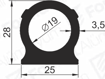
Pr.No: 1725 0,930 kg/m
