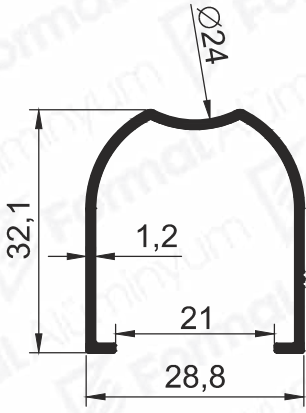
Pr.No: 1964 0,282 kg/m
