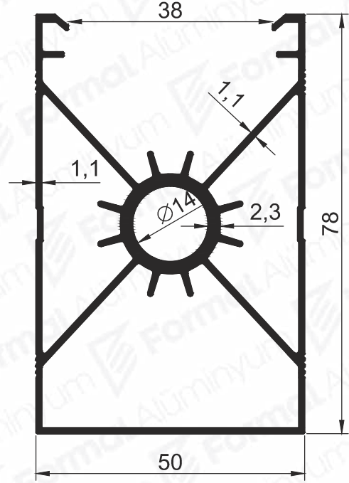
Pr.No: 1960 1,403 kg/m
