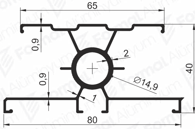
Pr.No: 8550 0,842 kg/m
