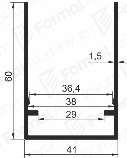
Pr.No: 8593 0,699 kg/m
