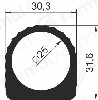
Pr.No: 8530 0,950 kg/m
