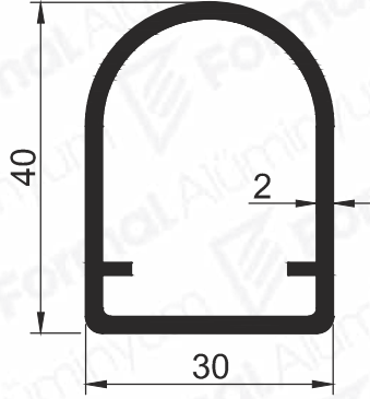
Pr.No: 8036 0,677 kg/m
