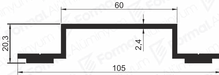
Pr.No: 1726 1,065 kg/m
