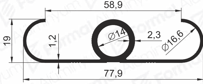
Pr.No: 1963 0,673 kg/m
