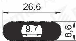
Pr.No: 8861 0,417 kg/m
