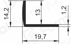
Pr.No: 9961 0,114 kg/m
