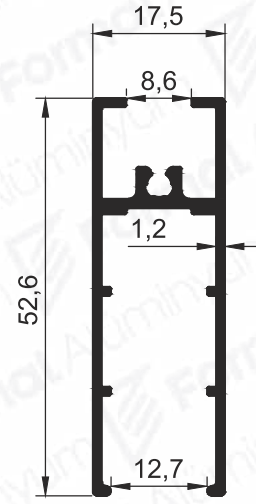
Pr.No: 9735 0,492 kg/m
