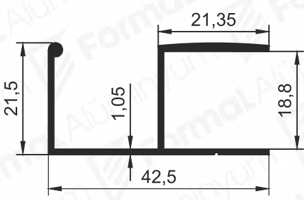
Pr.No: 1789 0,320 kg/m
