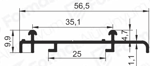
Pr.No:1472 0,290 Kg/m
