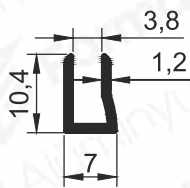
Pr.No: 1141 0,081 kg/m
