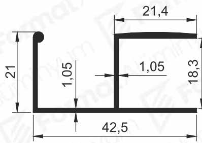
Pr.No: 9322 0,318 kg/m
