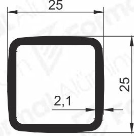
Pr.No: 9921 0,447 kg/m
