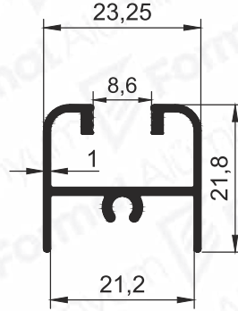
Pr.No: 1466 0,269 kg/m
