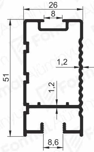
Pr.No: 9634 0,574 kg/m
