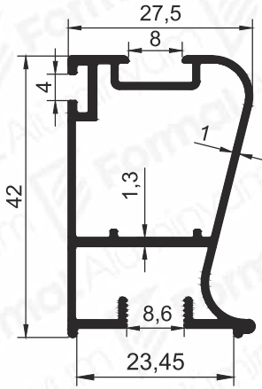
Pr.No: 1727 0,506 kg/m
