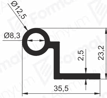
Pr.No: 9596 0,443 kg/m
