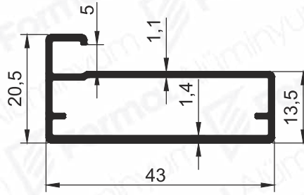
Pr.No: 9631 0,414 kg/m
