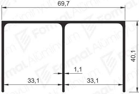
Pr.No: 8535 0,615 kg/m
