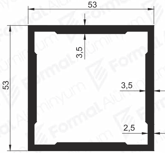
Pr.No: 1401 1,688 kg/m
