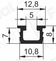
Pr.No: 9688 0,102 kg/m
