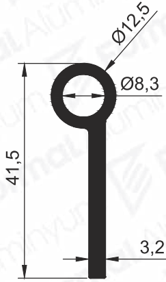
Pr.No: 9643 0,444 kg/m
