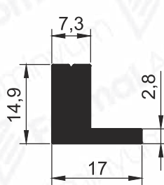
Pr.No: 9330 0,367 kg/m
