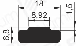
Pr.No: 9728 0,292 kg/m
