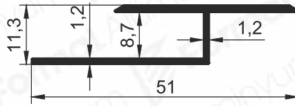
Pr.No: 2196 0,425 kg/m
