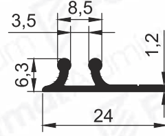
Pr.No: 9968 0,124 kg/m
