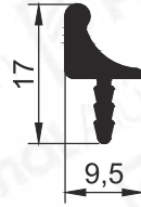
Pr.No: 1444 0,144 kg/m
