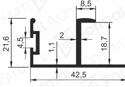
Pr.No: 1967 0,363 kg/m
