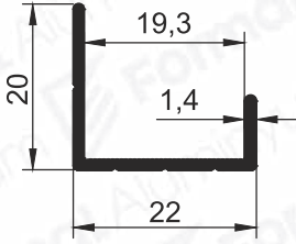
Pr.No: 1615 0,167 kg/m
