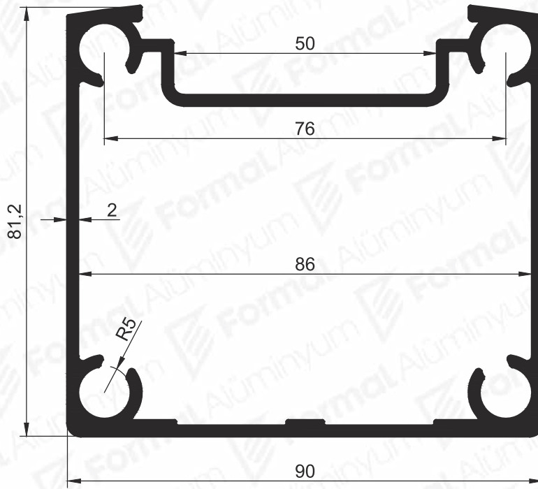
Pr.No: 9295 2,459 kg/m
