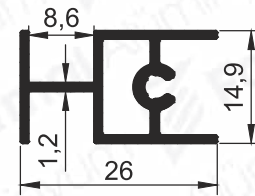
Pr.No: 5279 0,276 kg/m
