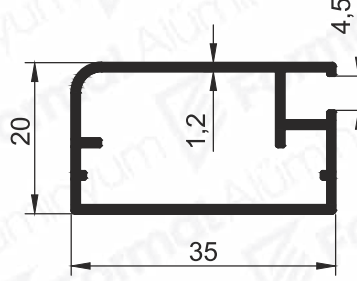
Pr.No: 9993 0,385 kg/m
