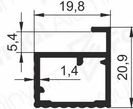
Pr.No: 9866 0,261 kg/m
