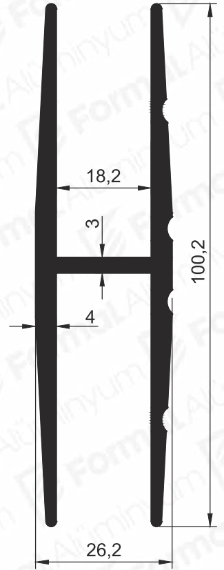
Pr.No: 9963 1,837 kg/m
