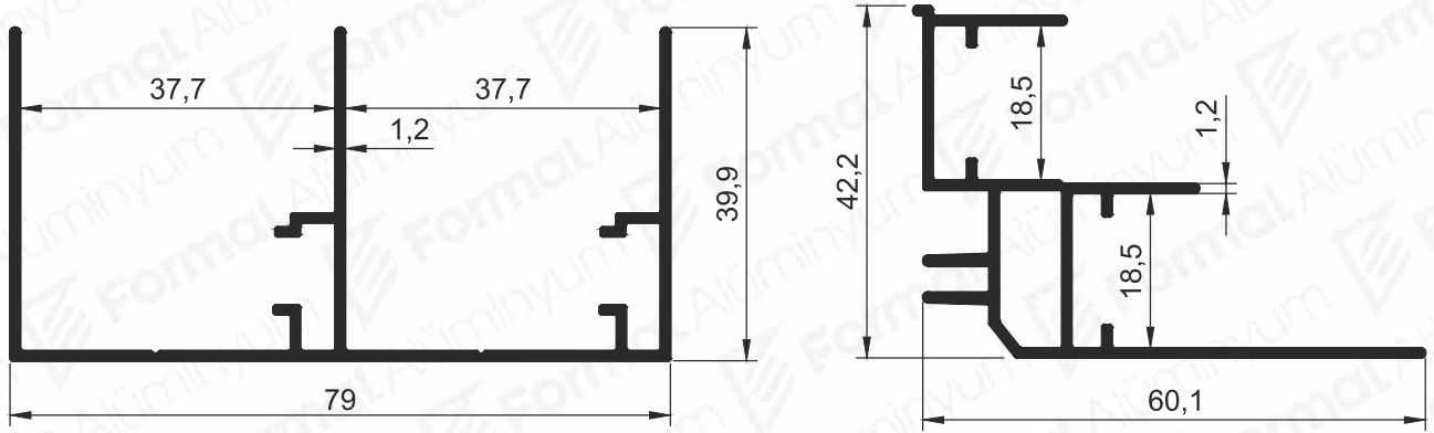
Pr.No: 4611 0,734 kg/m
