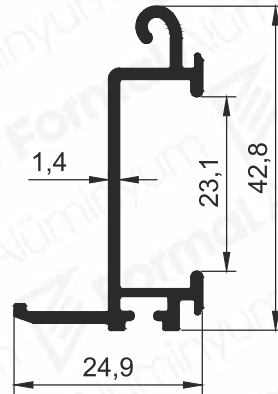
Pr.No: 1123 0,368 kg/m
