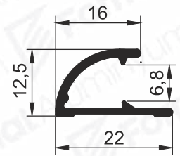
Pr.No: 1813 0,156 kg/m
