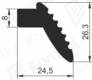
Pr.No: 8067 0,614 kg/m
