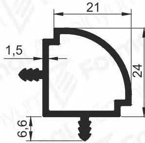
Pr.No: 9360 0,425 kg/m
