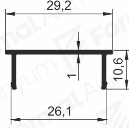
Pr.No: 9957 0,132 kg/m
