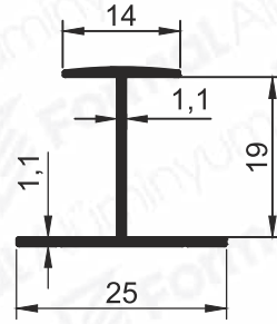
Pr.No: 4751 0,171 kg/m
