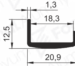
Pr.No: 8738 0,168 kg/m
