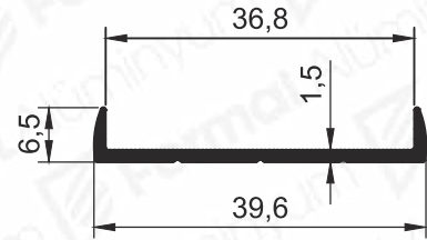
Pr.No: 1614 0,445 kg/m
