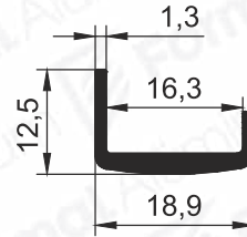
Pr.No: 8743 0,160 kg/m
