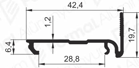
Pr.No: 9976 0,266 kg/m
