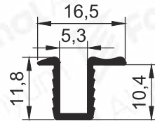
Pr.No: 1186 0,110 kg/m
