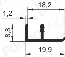
Pr.No: 9149 0,117 kg/m
