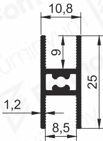
Pr.No: 1739 0,230 kg/m
