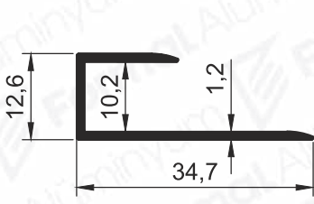
Pr.No: 2241 0,189 kg/m
