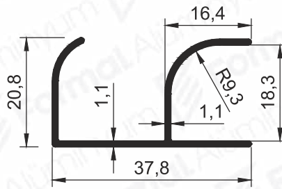
Pr.No: 8737 0,267 kg/m
