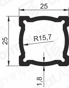
Pr.No: 1659 0,498 kg/m
