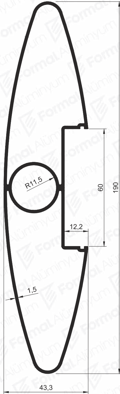
Pr.No: 1765 2,061 kg/m
