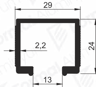
Pr.No: 8589 0,480 kg/m
