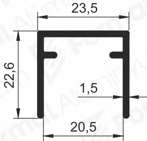
Pr.No: 9557 0,292 kg/m
