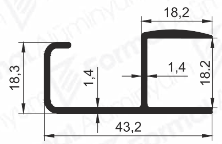
Pr.No: 8775 0,386 kg/m
