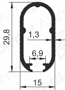
Pr.No: 1074 0,260 kg/m
