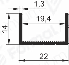
Pr.No: 1656 0,159 kg/m
