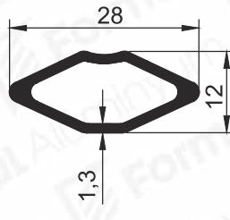
Pr.No: 8076 0,221 kg/m
