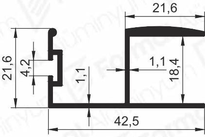
Pr.No: 9745 0,406 kg/m
