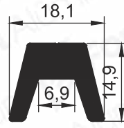
Pr.No: 9238 0,383 kg/m
