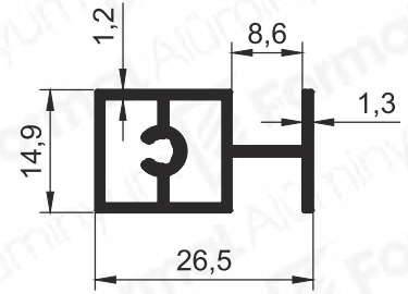
Pr.No: 1644 0,335 kg/m
