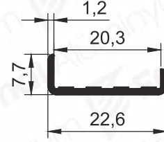
Pr.No: 9991 0,108 kg/m
