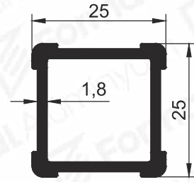
Pr.No: 9358 0,497 kg/m
