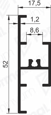
Pr.No: 9736 0,391 kg/m
