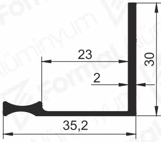
Pr.No: 1631 0,295 kg/m
