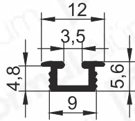
Pr.No: 1134 0,067 kg/m
