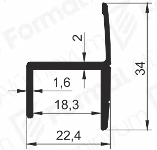
Pr.No: 1246 0,319 kg/m
