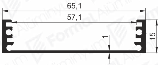
Pr.No: 2548 0,376 kg/m
