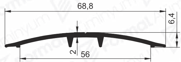
Pr.No: 1968 0,337 kg/m
