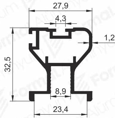
Pr.No: 8995 0,487 kg/m
