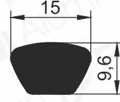
Pr.No: 9727 0,317 kg/m
