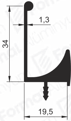
Pr.No: 9684 0,482 kg/m
