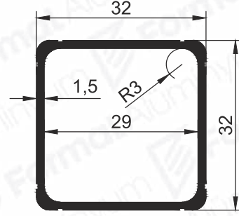
Pr.No: 3768 0,496 kg/m
