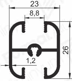
Pr.No: 8536 0,357 kg/m
