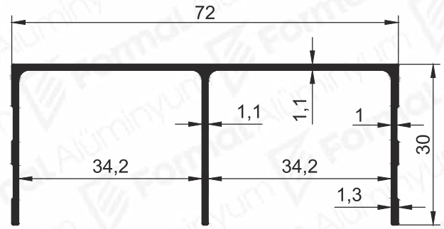
Pr.No:1470 0,493 Kg/m
