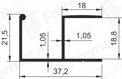
Pr.No: 3714 0,274 kg/m
