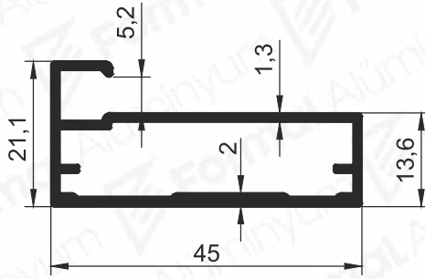
Pr.No: 9868 0,522 kg/m
