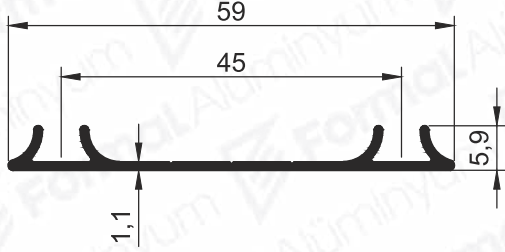
Pr.No: 9838 0,232 kg/m
