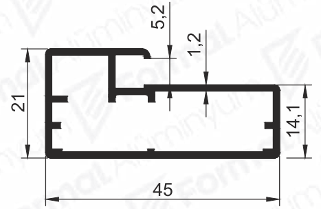
Pr.No: 8884 0,466 kg/m
