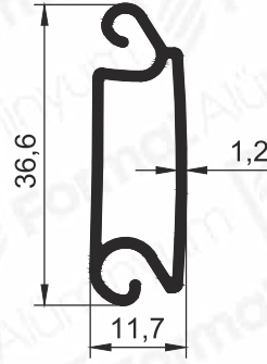
Pr.No: 9681 0,306 kg/m
