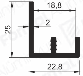
Pr.No: 2214 0,327 kg/m
