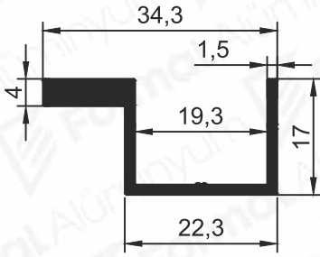
Pr.No: 1440 0,347 kg/m
