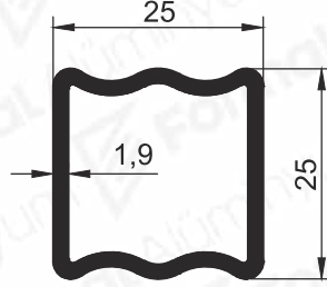
Pr.No: 9680 0,449 kg/m
