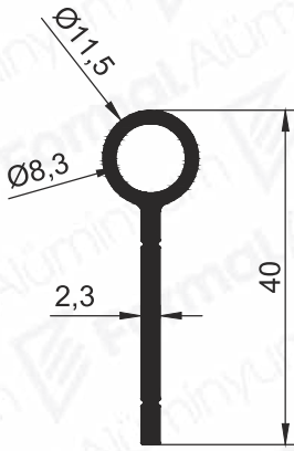
Pr.No: 2274 0,312 kg/m
