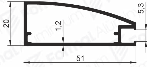
Pr.No: 9962 0,464 kg/m
