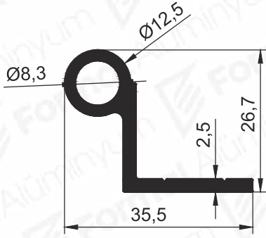
Pr.No: 9595 0,466 kg/m
