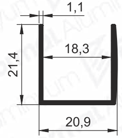
Pr.No: 1257 0,192 kg/m
