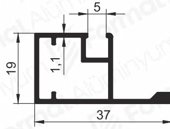
Pr.No: 1810 0,333 kg/m
