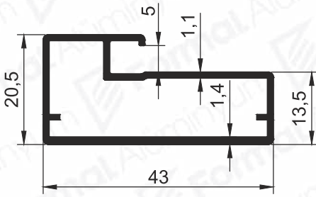
Pr.No: 9630 0,430 kg/m
