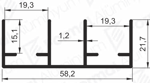
Pr.No: 9288 0,520 kg/m
