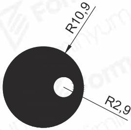
Pr.No: 8594 0,943 kg/m
