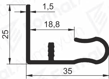
Pr.No: 8769 0,360 kg/m
