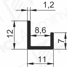
Pr.No: 9706 0,089 kg/m
