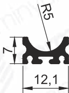
Pr.No: 1075 0,108 kg/m
