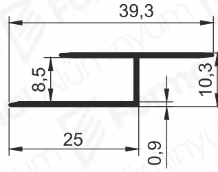
Pr.No: 8968 0,149 kg/m
