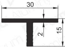
Pr.No: 8730 0,273 kg/m
