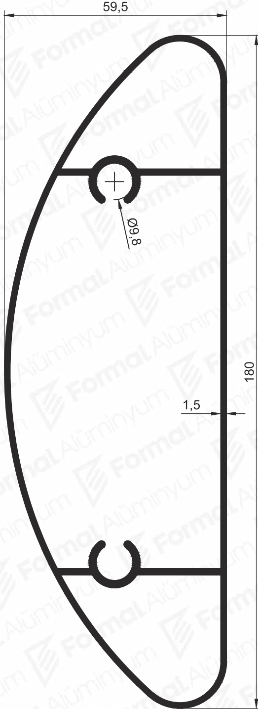
Pr.No: 1117 2,260 kg/m
