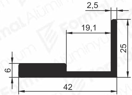
Pr.No: 1474 0,627 kg/m
