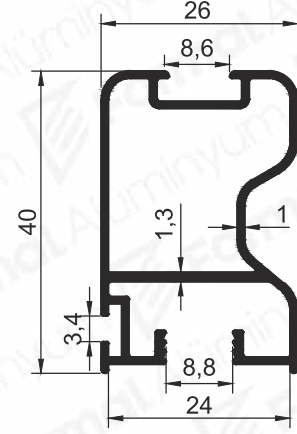
Pr.No: 1806 0,467 kg/m
