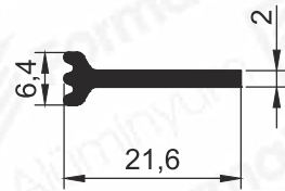
Pr.No: 8105 0,141 kg/m
