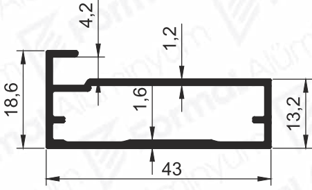
Pr.No: 9832 0,418 kg/m
