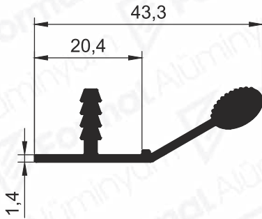
Pr.No: 2805 0,390 kg/m
