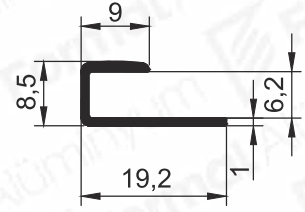
Pr.No: 9348 0,097 kg/m
