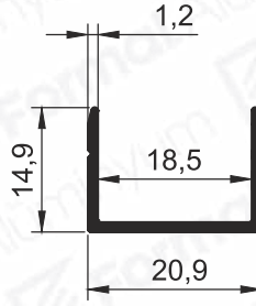
Pr.No: 8846 0,154 kg/m
