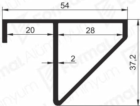
Pr.No: 2715 0,658 kg/m
