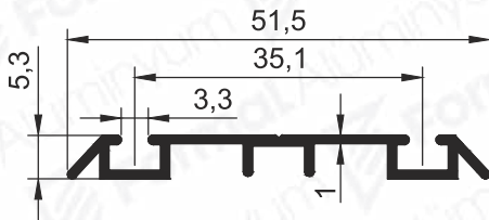
Pr.No:1471 0,243 kg/m
