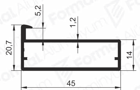
Pr.No: 1851 0,423 kg/m
