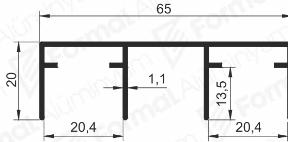
Pr.No: 9686 0,458 kg/m
