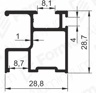
Pr.No: 1641 0,417 kg/m
