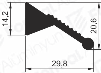
Pr.No: 8071 0,459 kg/m
