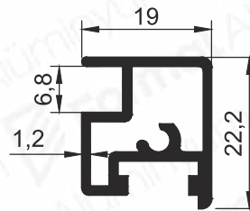
Pr.No: 8754 0,355 kg/m
