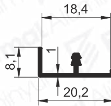
Pr.No: 9719 0,102 kg/m
