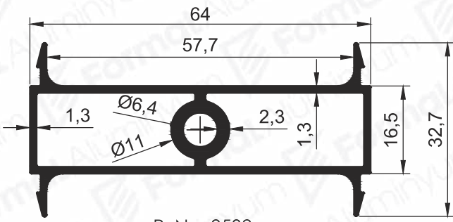
Pr.No: 9532 0,865kg/m
