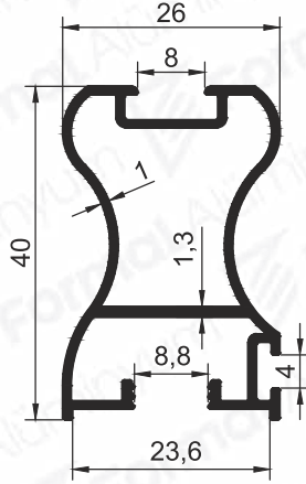
Pr.No: 2233 0,452 kg/m
