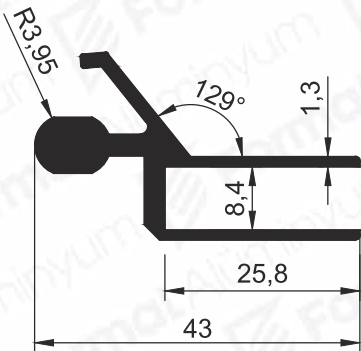
Pr.No: 1170 0,578 kg/m
