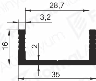
Pr.No: 8774 0,409 kg/m
