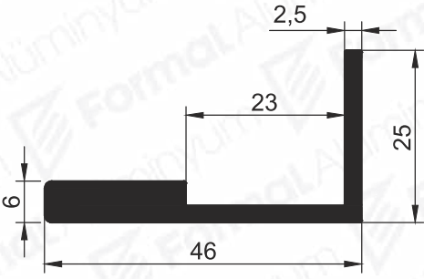
Pr.No: 1496 0,657 kg/m
