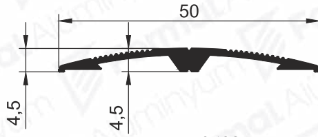
Pr.No: 9428 0,213 kg/m
