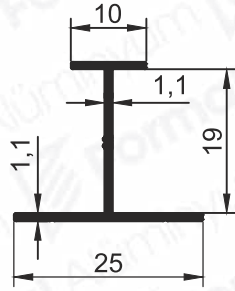
Pr.No: 1439 0,158 kg/m
