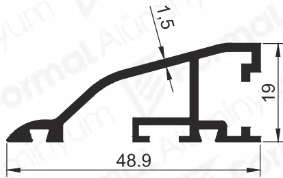
Pr.No: 8103 0,463 kg/m
