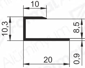
Pr.No: 8967 0,092 kg/m
