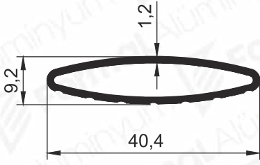
Pr.No: 9787 0,262 kg/m
