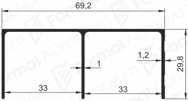
Pr.No: 9624 0,440 kg/m
