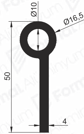
Pr.No: 9635 0,737 kg/m
