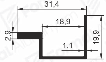
Pr.No: 1630 0,240 kg/m
