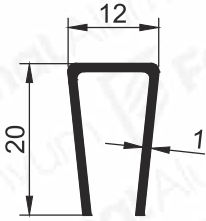
Pr.No: 9109 0,136 kg/m
