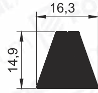
Pr.No: 9239 0,489 kg/m
