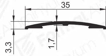
Pr.No: 9443 0,120 kg/m
