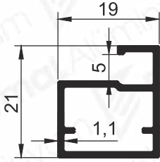
Pr.No: 9629 0,239 kg/m
