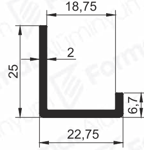
Pr.No: 2428 0,272 kg/m
