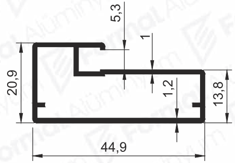
Pr.No: 8866 0,413 kg/m
