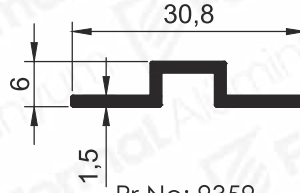
Pr.No: 9359 0,162 kg/m
