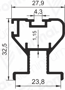
Pr.No: 1750 0,432 kg/m
