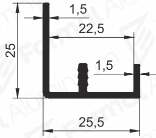
Pr.No: 1497 0,273 kg/m
