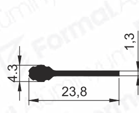
Pr.No: 8081 0,118 kg/m
