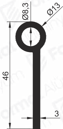
Pr.No: 9636 0,486 kg/m
