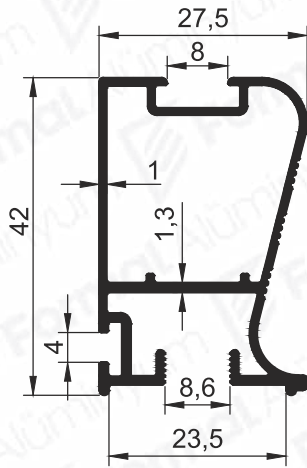
Pr.No: 9718 0,498 kg/m
