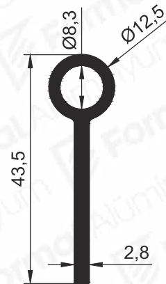
Pr.No: 9637 0,428 kg/m
