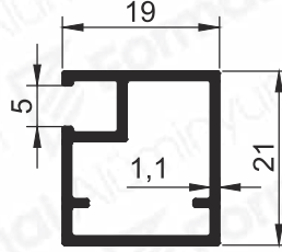
Pr.No: 9627 0,261 kg/m
