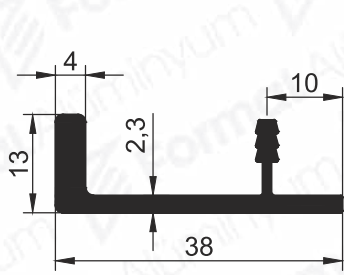
Pr.No: 2786 0,406 kg/m
