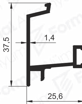
Pr.No: 8911 0,343 kg/m
