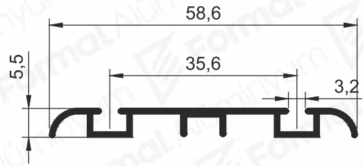
Pr.No: 8534 0,274 kg/m
