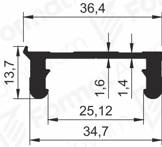
Pr.No: 1480 0,380 kg/m
