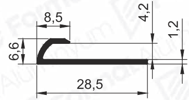
Pr.No: 1028 0,127 kg/m
