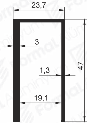
Pr.No:1200 0,616 kg/m
