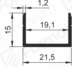
Pr.No: 1601 0,155 kg/m
