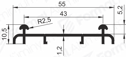
Pr.No: 9687 0,323 kg/m
