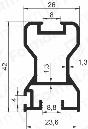
Pr.No: 8540 0,585 kg/m
