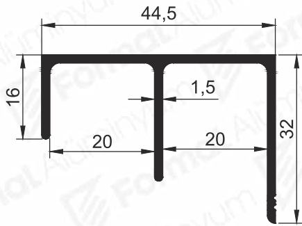
Pr.No: 8108 0,459 kg/m
